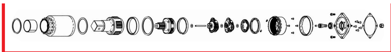
Vue éclatée d'une boîte de vitesses RAD
